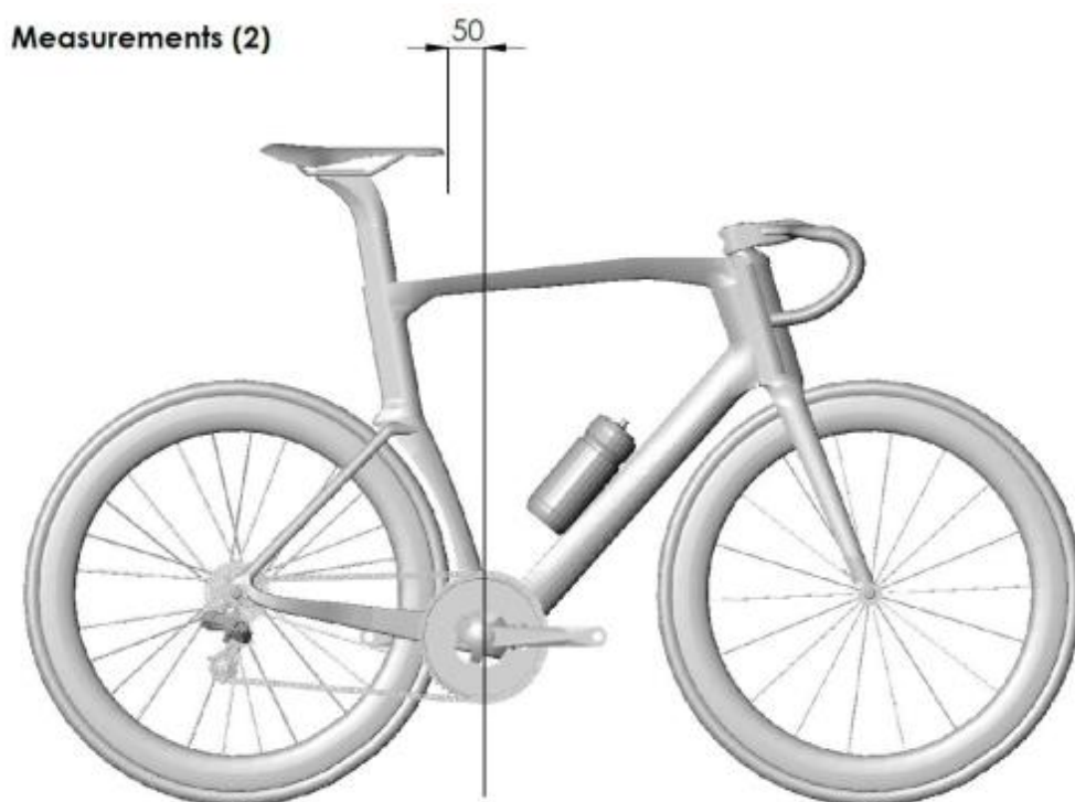
rysunek „Wymiary (2)”
